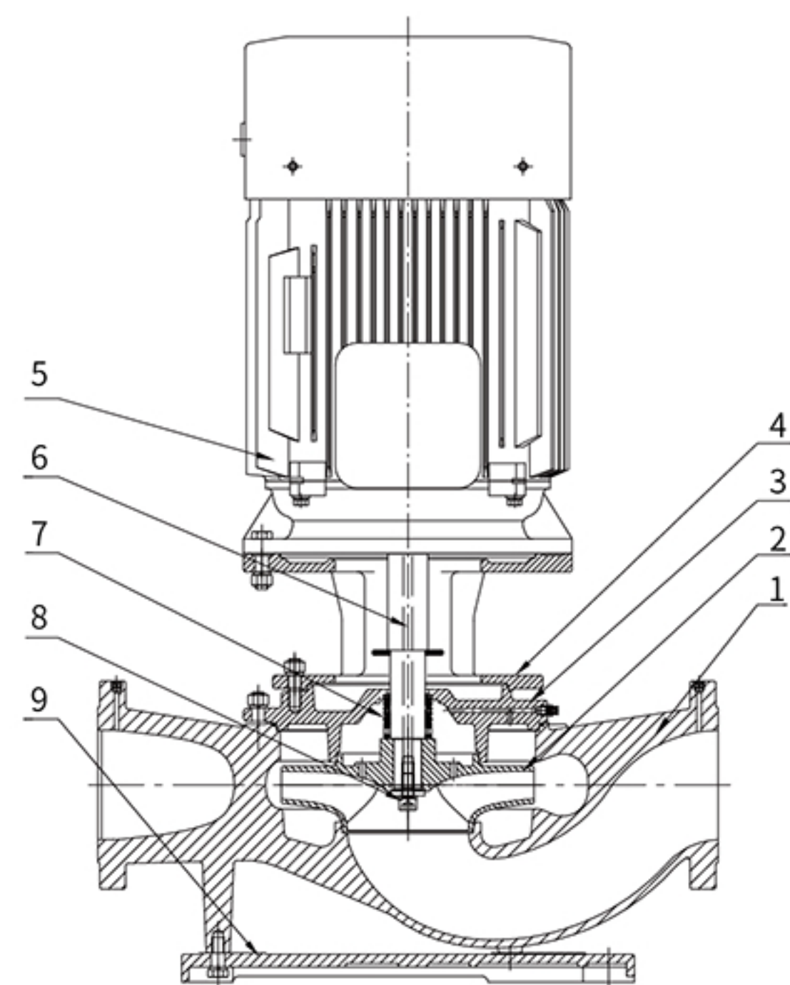
● SLZ结构图 SLZ Structure Drawing
