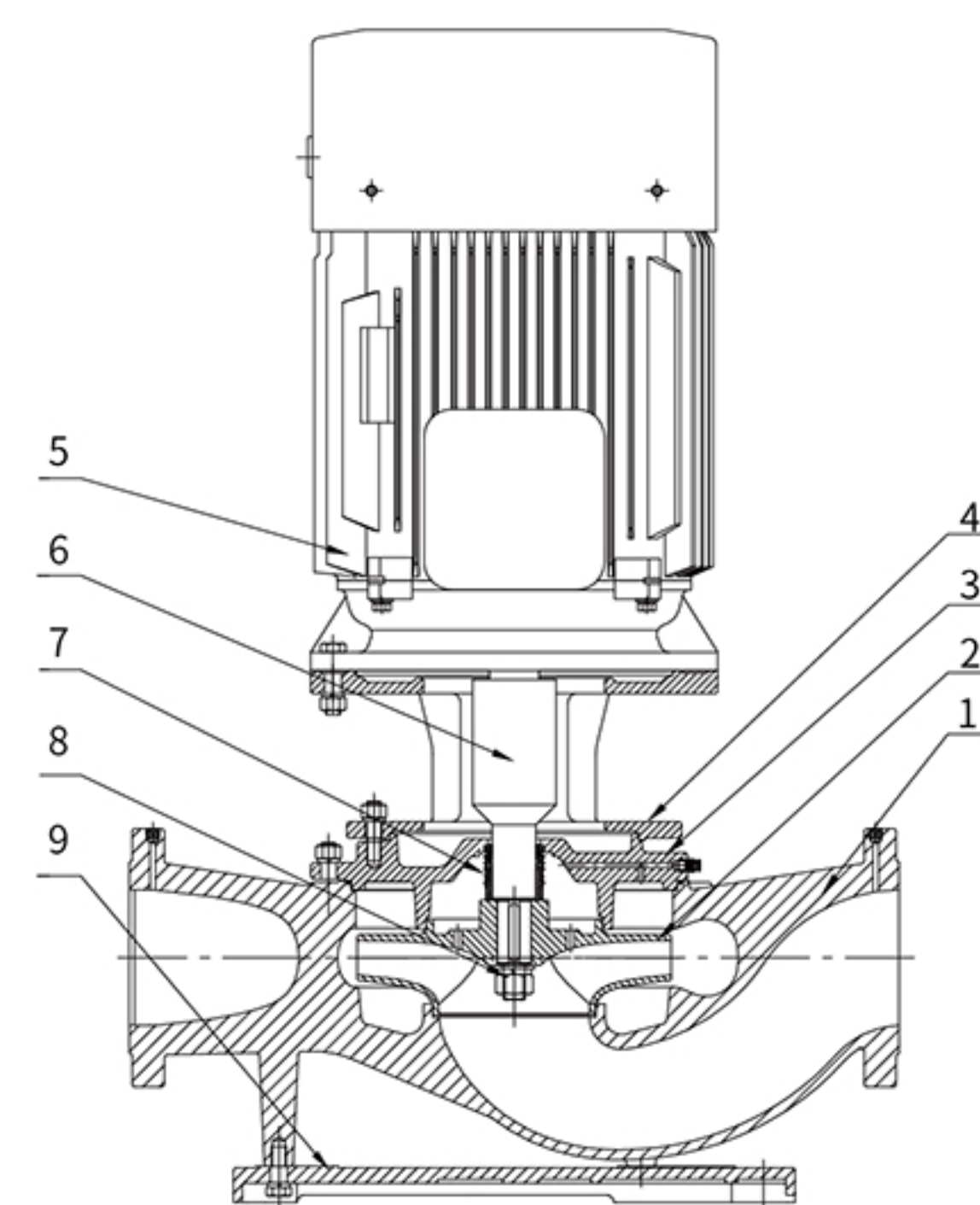
● SL结构图 SL Structure Drawing
