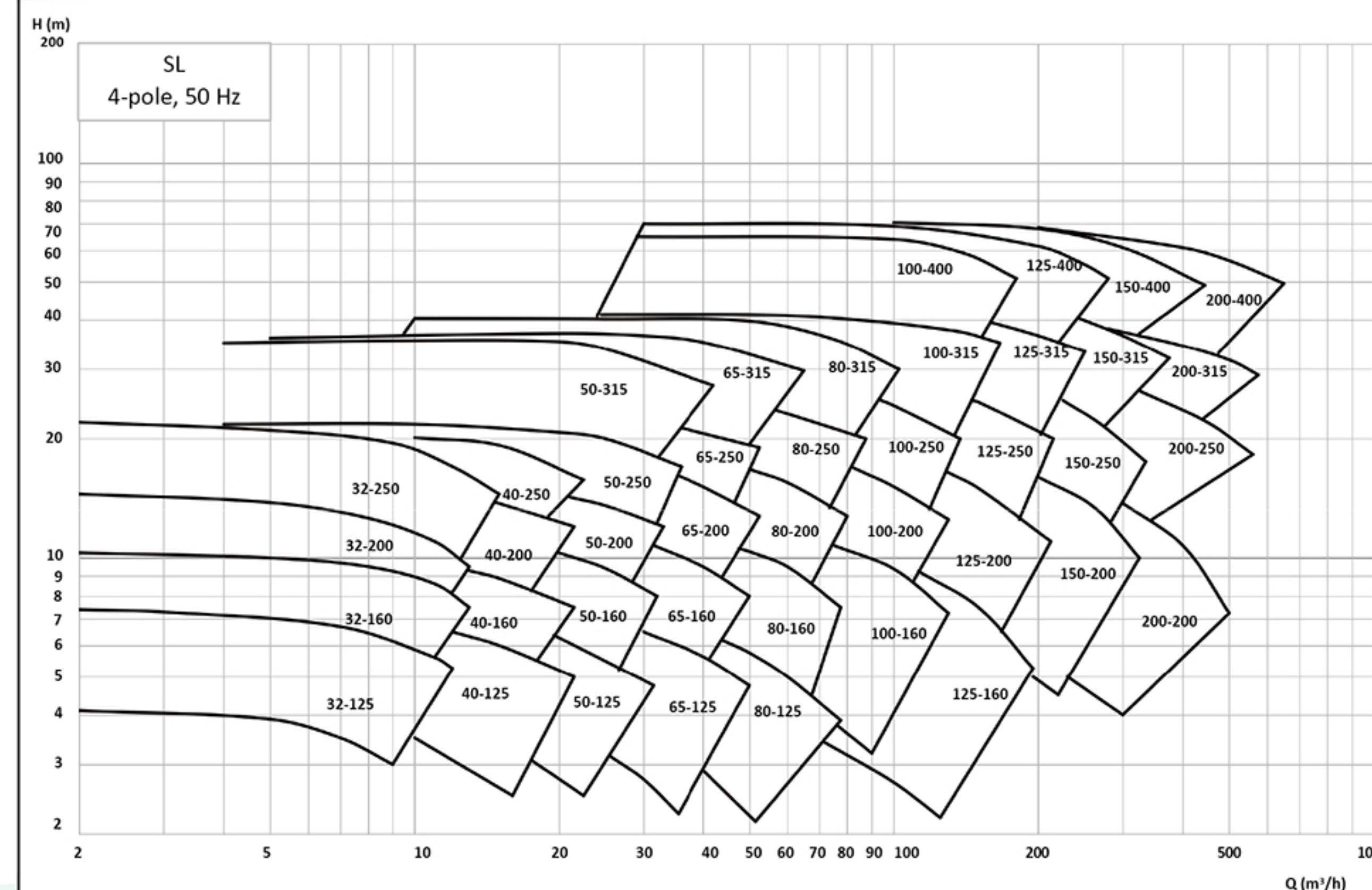
SL (Z) 4极 SL (Z) 4-Pole
